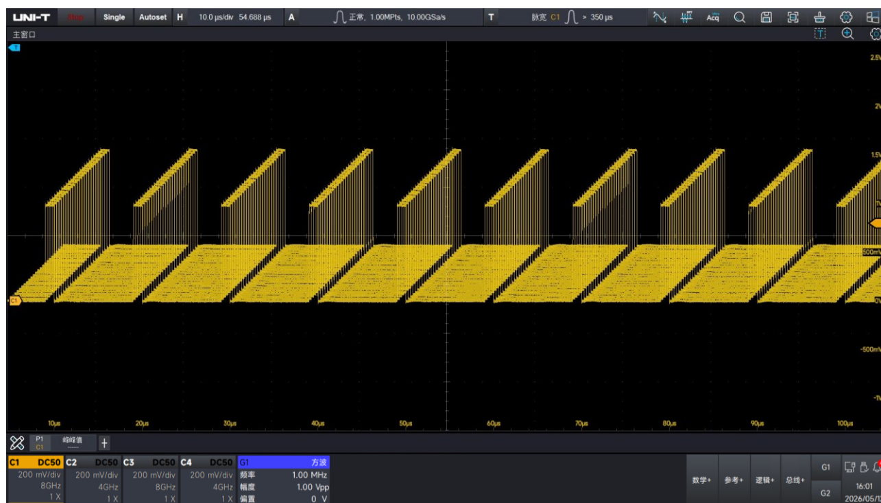
通过顺序模式同时查看多帧数据并以 45°显示
