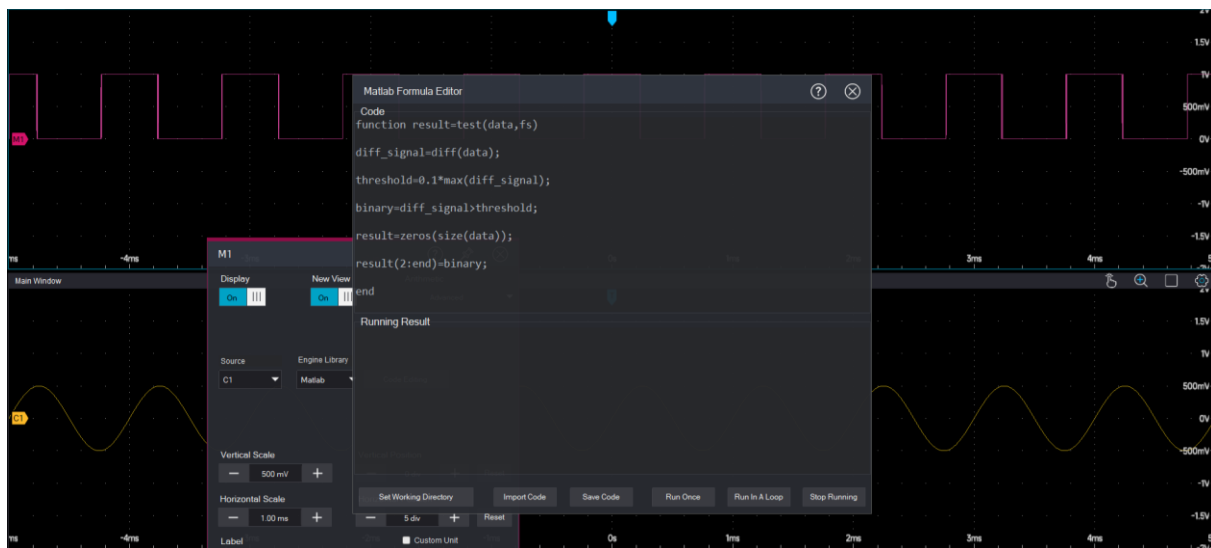
上图运用 matlab 脚本对通道 1 的正弦波进行差分处理，随后转化成方波
